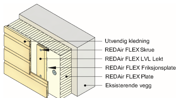
Fig. 1 Prinsipiell utførelse av ROCKWOOL REDAir FLEX monteret på eksisterende veggkonstruksjon. Eksempel med utvendig trekledning
