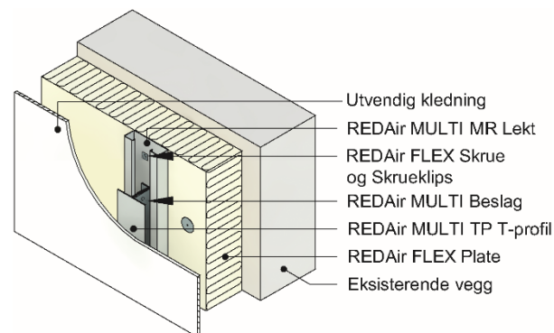
Fig. 2 Prinsipiell utførelse av ROCKWOOL REDAir MULTI monteret på eksisterende veggkonstruksjon. Eksempel med utvendig platekledning
